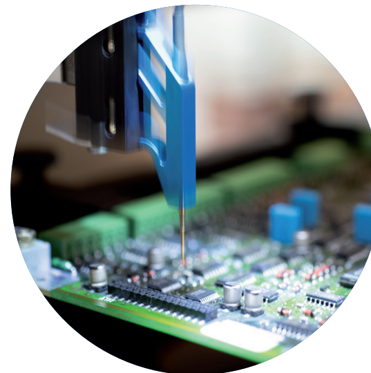
Das GRS550 besitzt eine moderne Schrittmotorsteuerung mit Überwachung aller Achsen per Encoder
