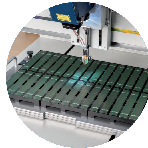
Bis zu 30 Testcoupons können in die Couponaufnahme eingelegt werden.
