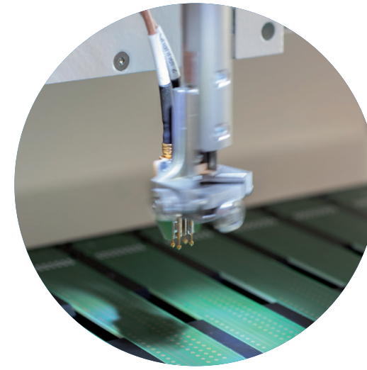
Das RITS 550 misst sowohl unsymmetrische als auch differentielle Impedanzen mittels einer neu konstruierten, drehbaren Prüfspitze.
