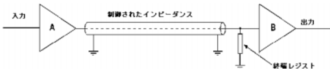
図 1 - シングル・エンド PCB トレース
