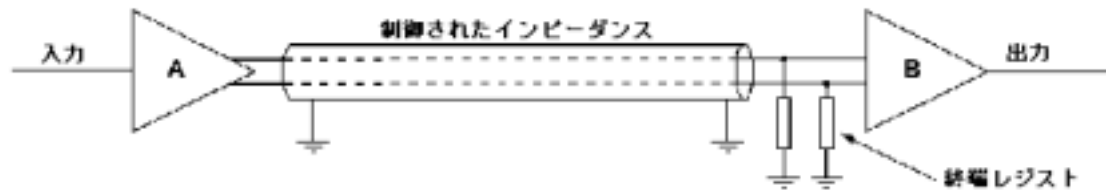
図2 - 差動プリント配線板トレース
